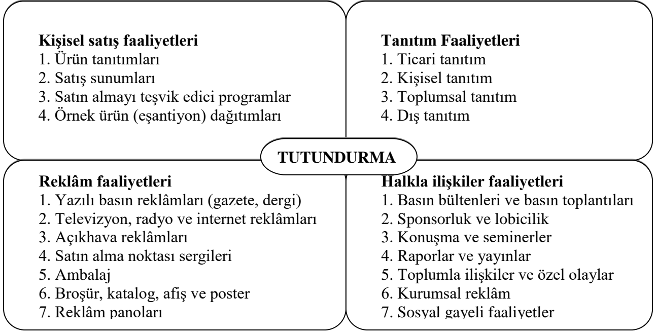
Şekil 9-6: Tutundurma Karması
